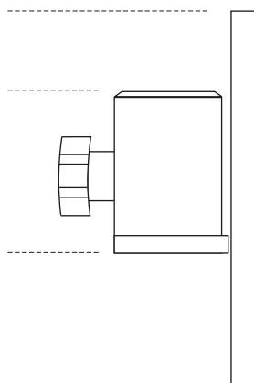
Sistema di ancoraggio a parete tramite tasselli da muro e viti a vista. Wall anchoring system with wall anchors and exposed screws.
