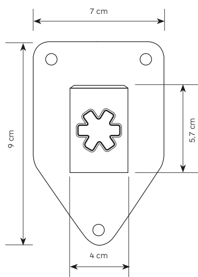
Sistema di ancoraggio a parete tramite tasselli da muro e viti a vista. Wall anchoring system with wall anchors and exposed screws.
